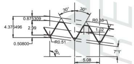
TAPER 1:4, 5 TPI V-040
