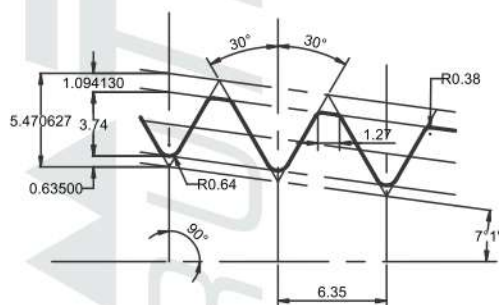
TAPER 1:4, 4 TPI V-050
