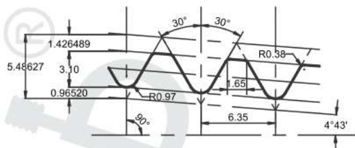
TAPER 1:6, 4 TPI V-038R
